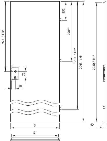
Rys. 2. Skrzydło przylgowe - wymiary.
