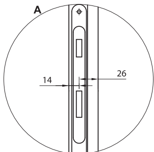
Rys. 1. Rozstaw wkładki w skrzydle
