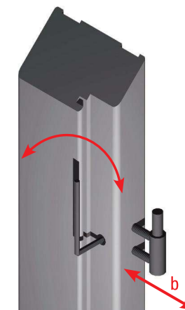
Rys. 3b regulacja zawiasu w ościeżnicy
